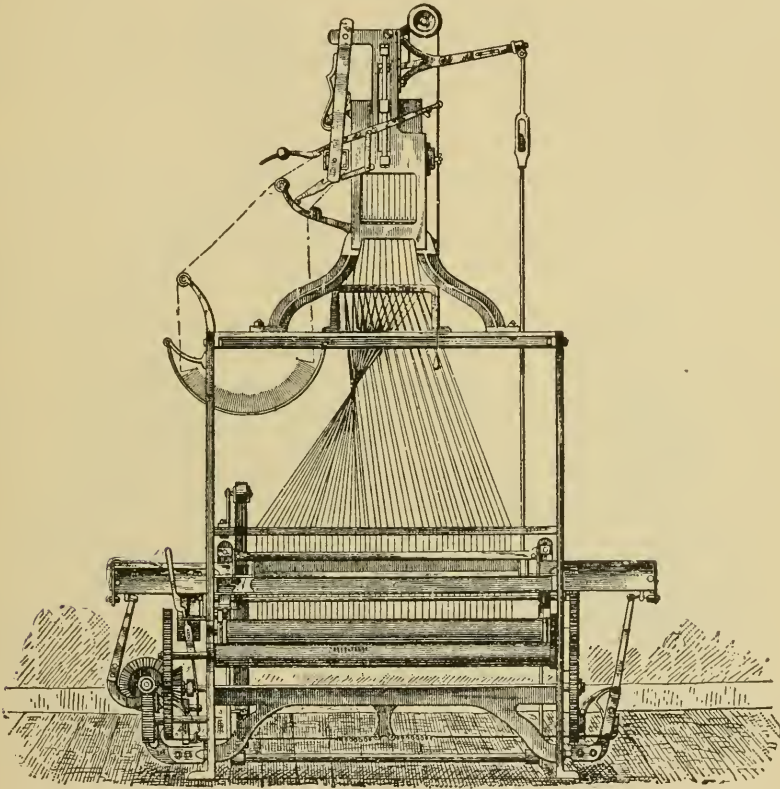
JACQUARD MACHINE.
